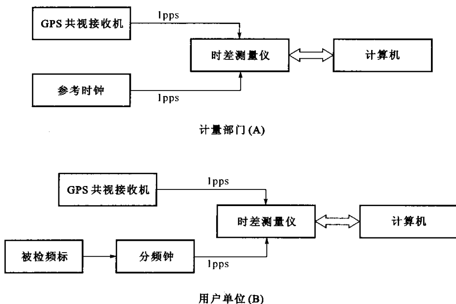
图 6 GPS 共视法校频
