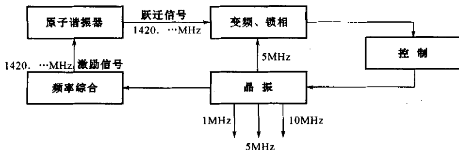
图 2 被动型氢原子频标
