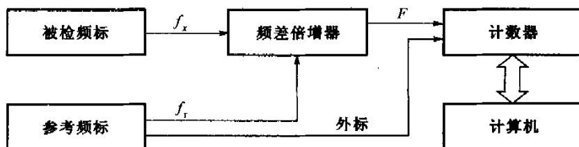
图 4 频率稳定度测量
