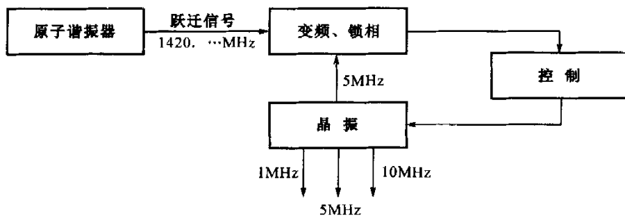
图 1 主动型氢原子频标
