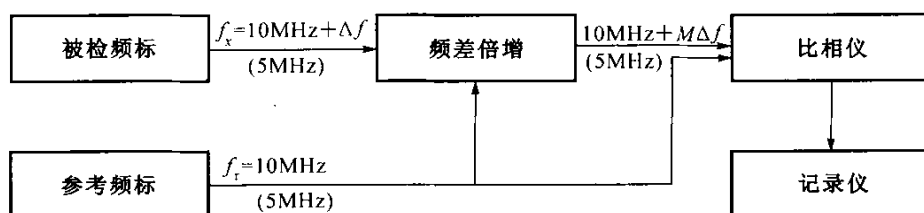
图 5 频率漂移、准确度及稳定度测量
